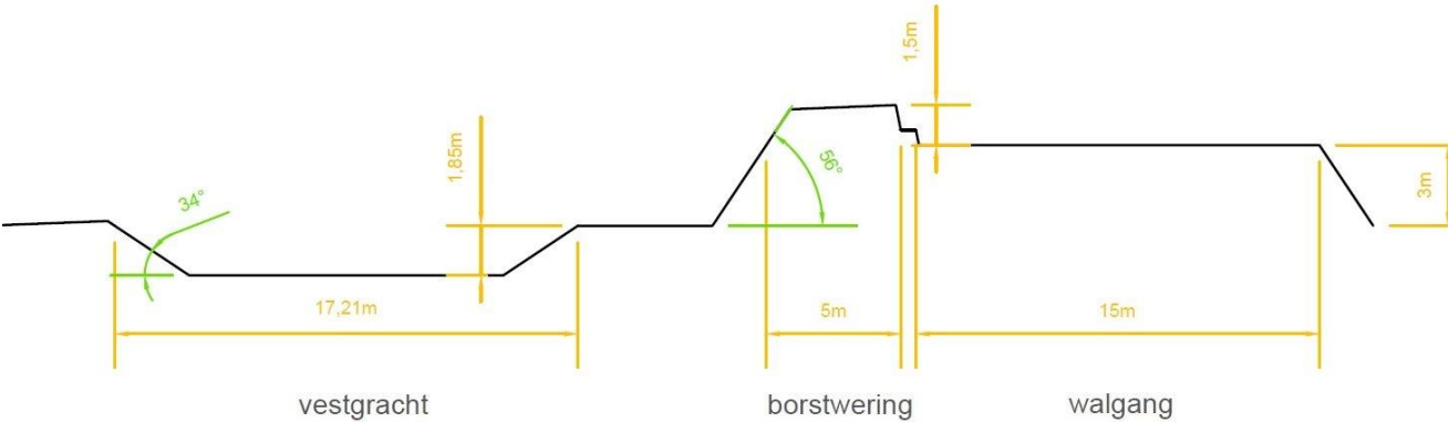
Dwarsdoorsnede stadswalling Herentals
